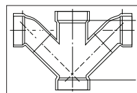
WYE de doble combinación/ curva de 1/8 SI
